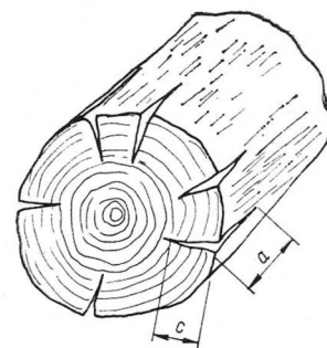
trhlina_měření.jpg
