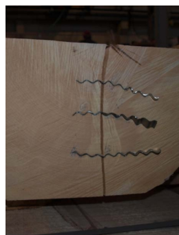
trhlina_drenova_svorky.jpg
